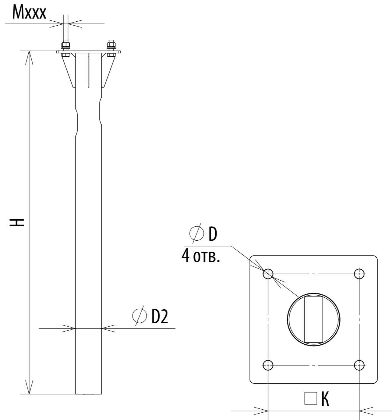
ОПТ4- Опора подземная трубная
