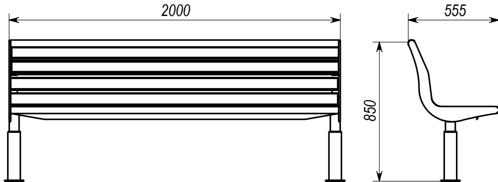
СК52 Скамейка Стрит ПМ-5-АФ-L2000-без подлокотников
