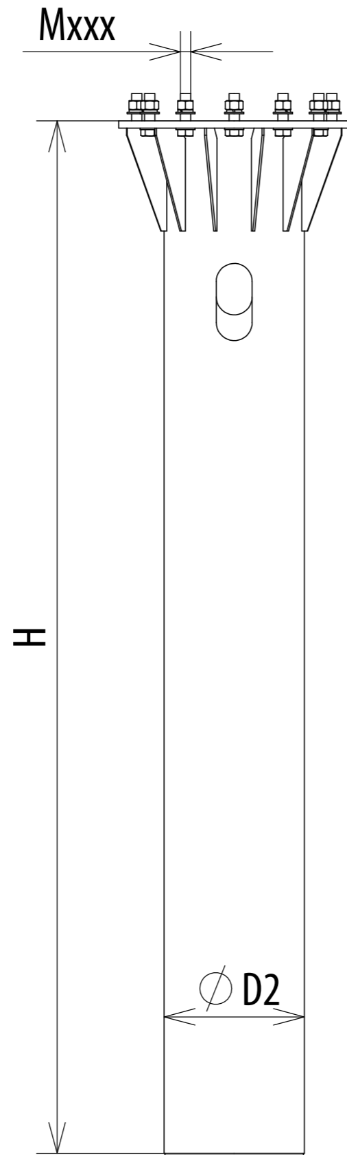
ОПТ12-Опора подземная трубная
