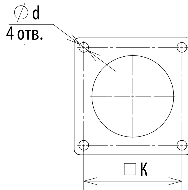
Фланец
