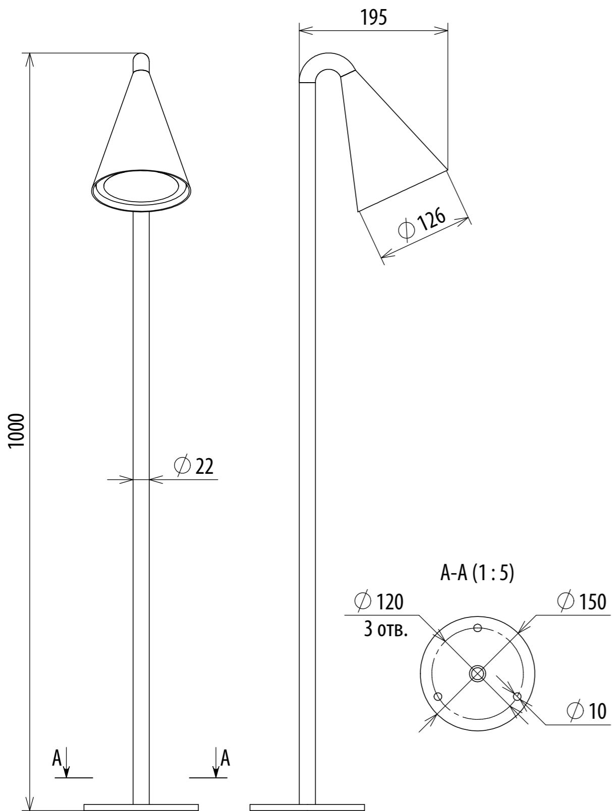
Сонетт мини ДТУ-170-АF-6Вт-1,0-1
