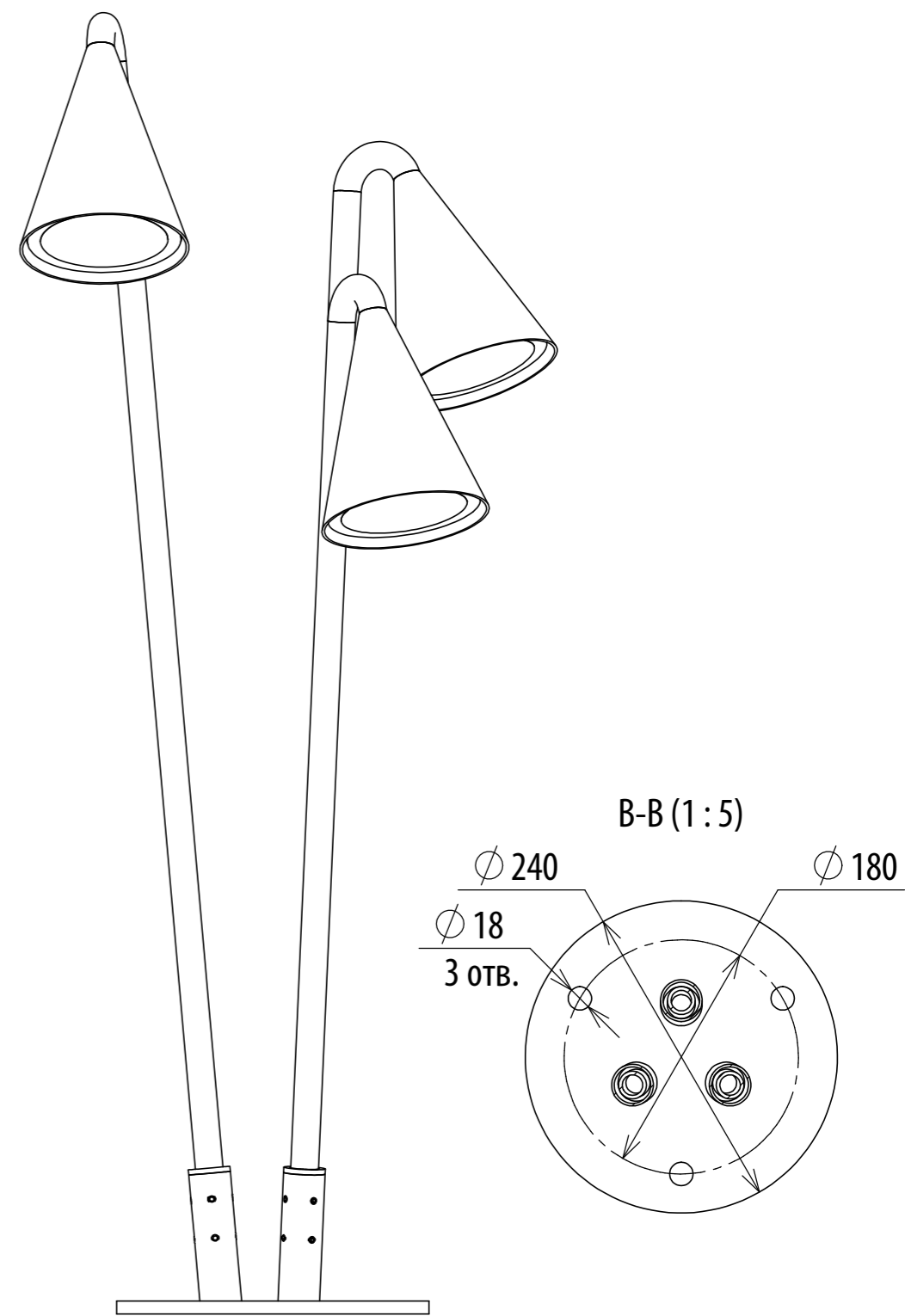
Сонетт мини ДТУ-170-АF-18Вт-1,0-3
