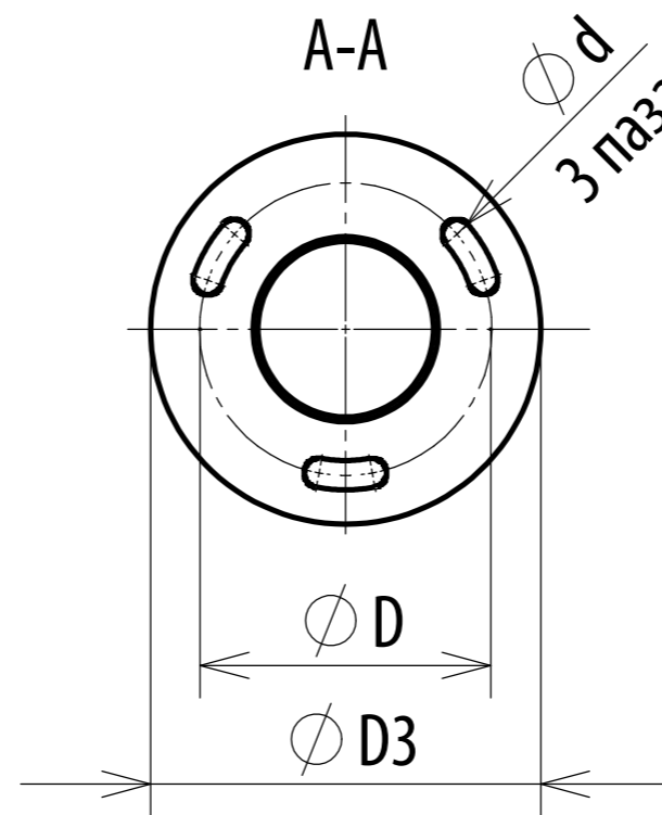
Фланец
