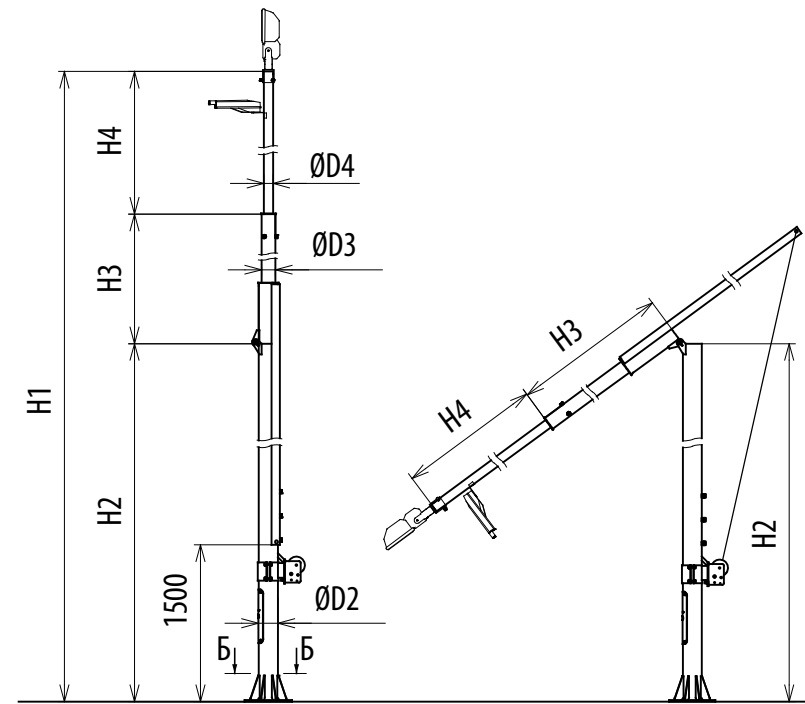
Опора СТО 10,0 - 14,0
