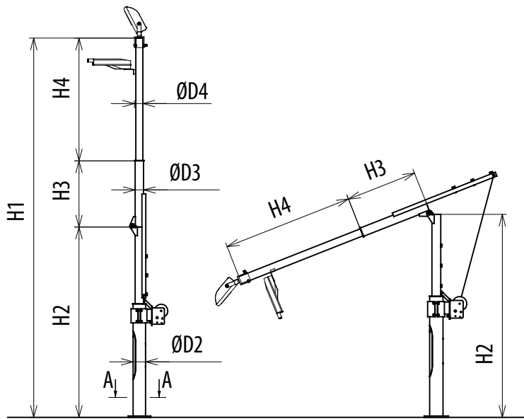
Опора СТО 3,6-9,0
