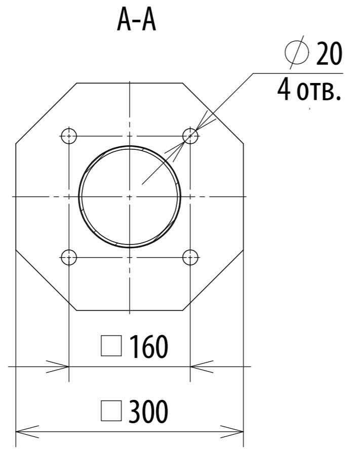
Фланец
