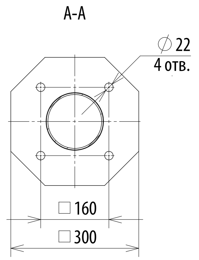
Фланец
